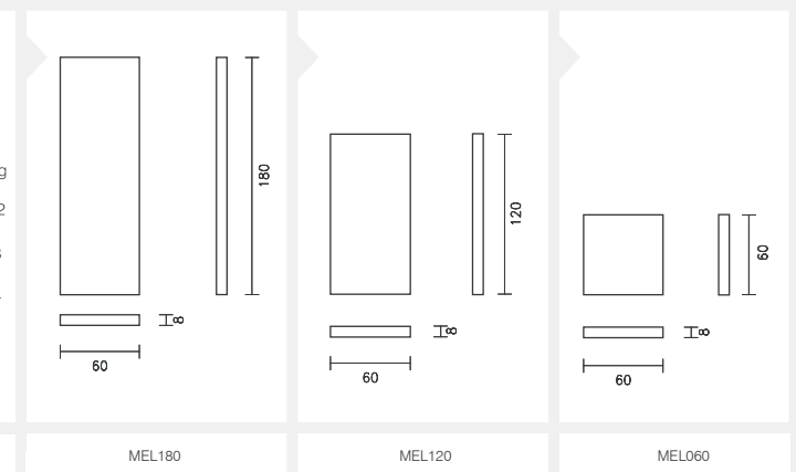
Desenhos técnicos
